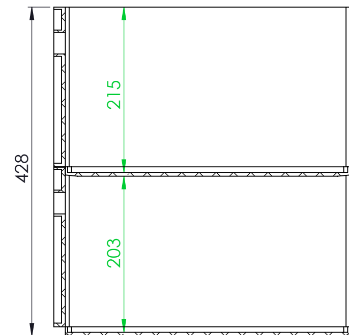
CUT A-A
