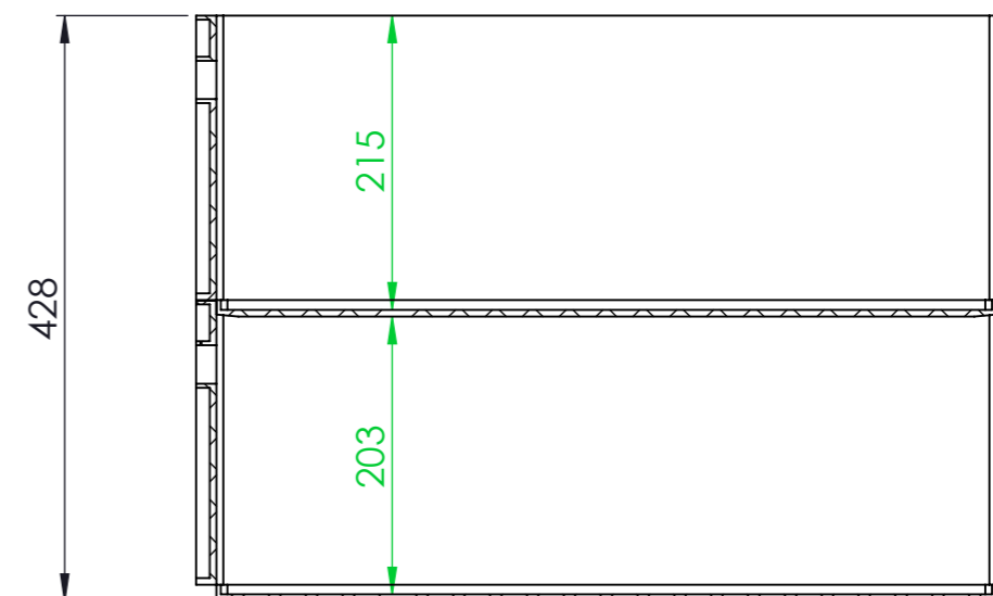
CUT A-A SCALE 1 : 6
