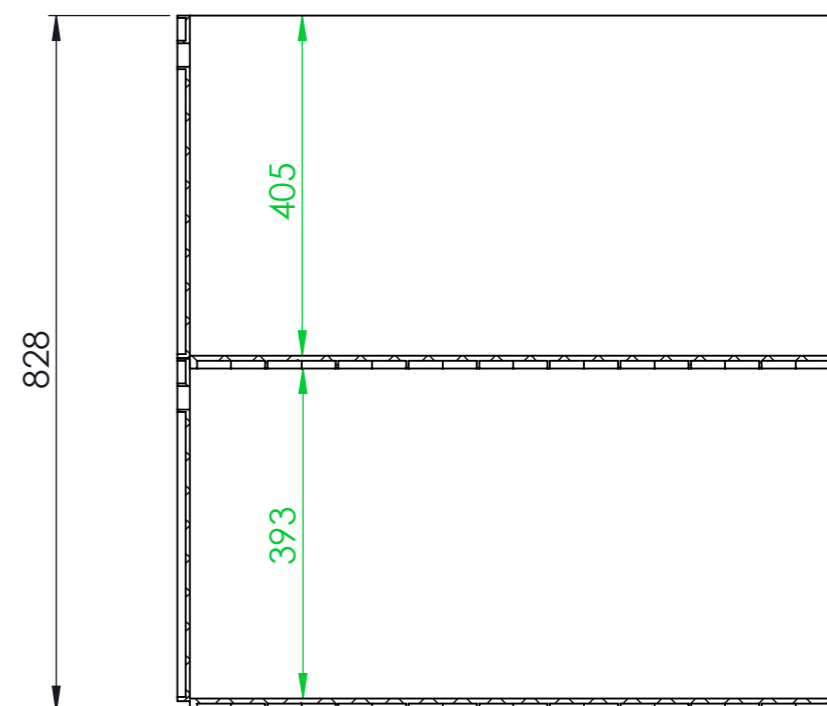
CUT A-A SCALE 1 : 9
